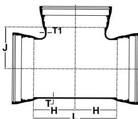
Tee
