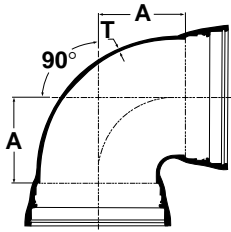
90° Bend
