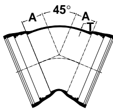
45° Bend
