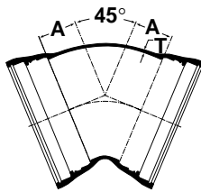
45° Bend
