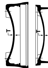
Cap Plug
