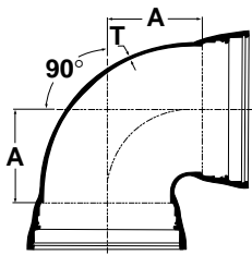
90° Bend
