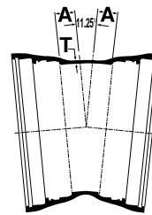
11 1/4° Bend
